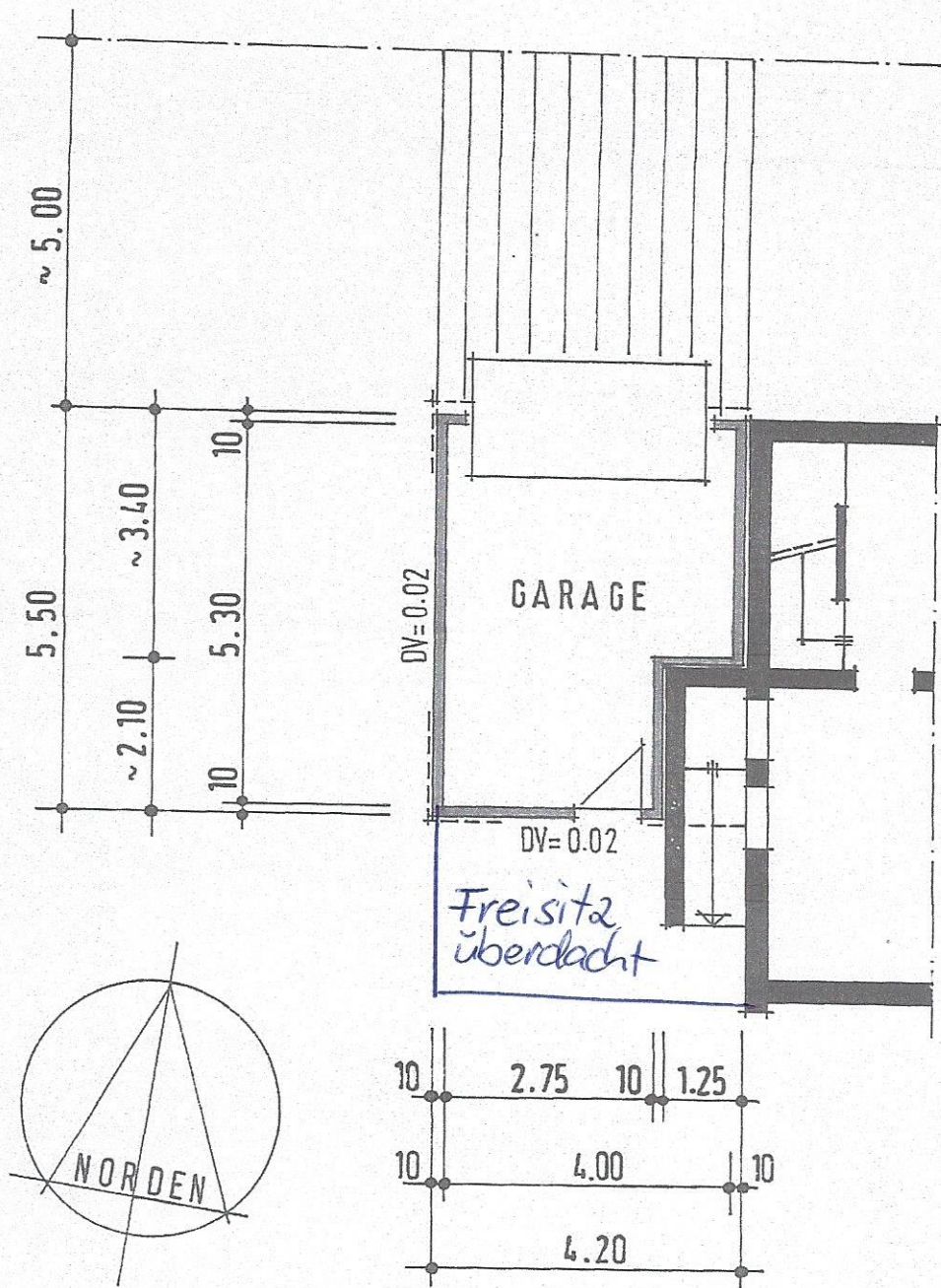
GRUNDRISS
