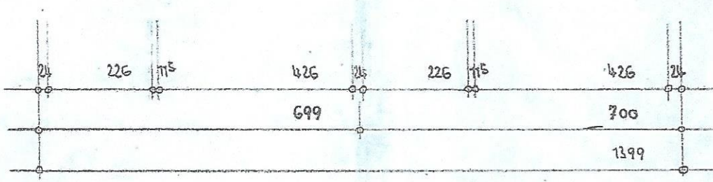
GRUNDRISS OBERGESCHOSS MASST. 1:100
